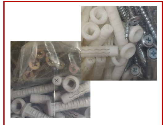
Schrauben mit Unyco™ Nylonanker mit abgerundetem Rand
